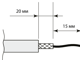
Рисунок 2. Зачистить кабель согласно рисунку.
