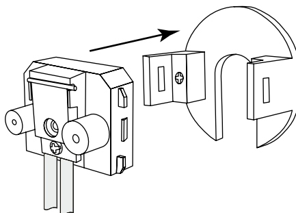
Рисунок 6. Вставить в суппорт электрическую часть розетки.
