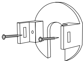
Рисунок 5. Суппорт закрепить шурупами на стене.
